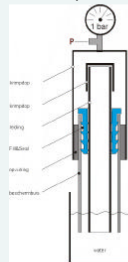
VMW test-opstelling
